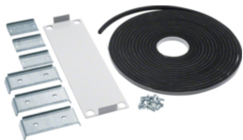
univers Zestaw łączeniowy gł. 400mm kl II
