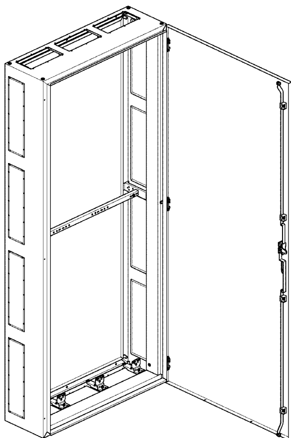
Rozdzielnica IP41 stojąca, głęb. 275 mm
