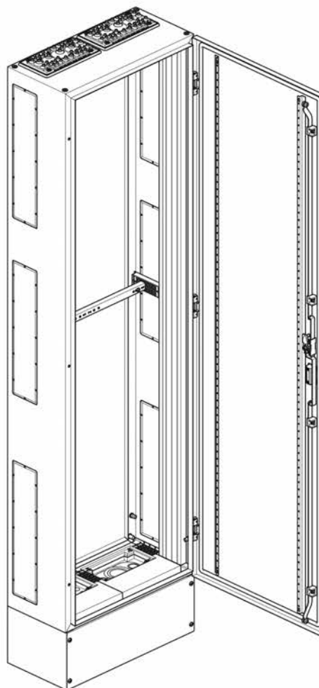
Rozdzielnica IP55 stojąca, głęb. 275 mm
