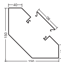
Profil trójkątny BRSS1501501EK
