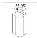
Narożnik zewnętrzny regulowany PC-ABS
