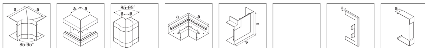
Narożnik wewnętrzny regulowany PC-ABS
