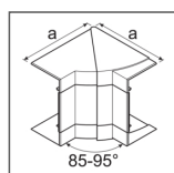
Narożnik wewnętrzny regulowany PC-ABS
