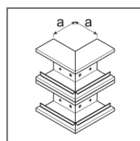
Narożnik zewnętrzny blacha stalowa
